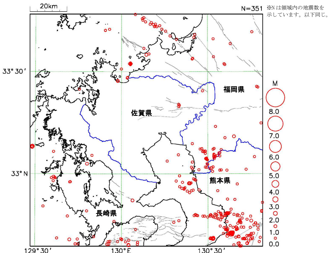
図 1 震央分布図 (2024 年 10 月 1 日～31 日、深さ 30km 以浅、M ≥ 0.0) 灰色の線は地震調査研究推進本部の長期評価による活断層を示しています。
