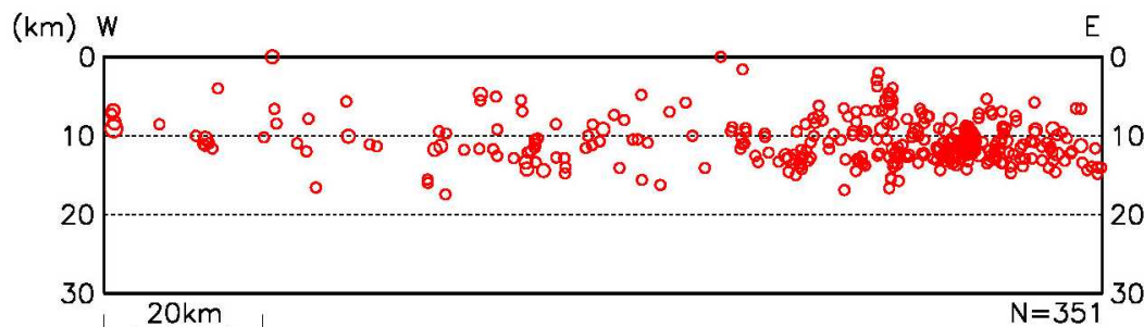
図 2 断面図 (2024 年 10 月 1 日～31 日、深さ 30km 以浅) 震央分布図を南の方から見た断面図です。
