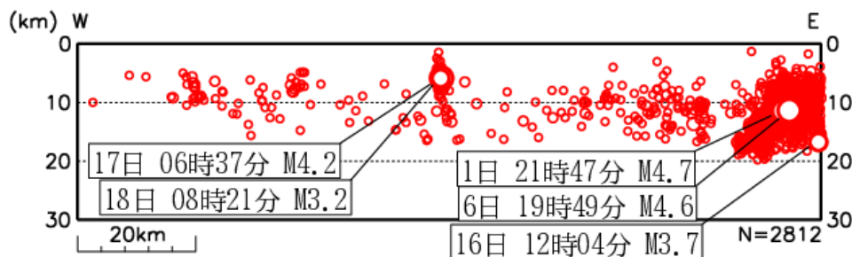
図 2 断面図 (2026 年 8 月 1 日～31 日、深さ 30km 以浅) 震央分布図を南の方から見た断面図です。
