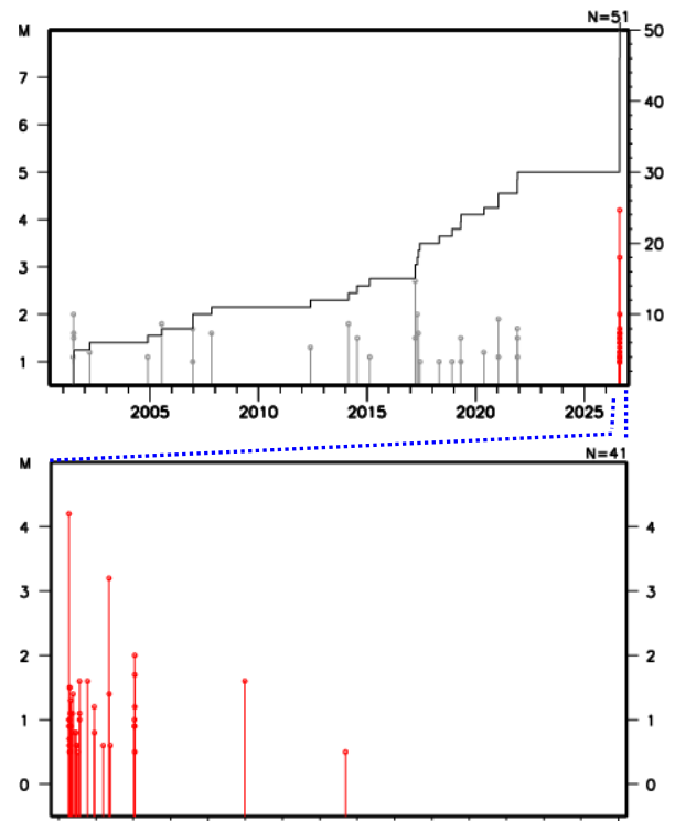
図12 図11の領域d内の地震活動経過図及び回数積算図
