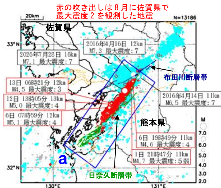
図4 震央分布図
