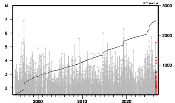
図 9 図 8 の領域 c 内の地震活動経過図及び回数積算図
