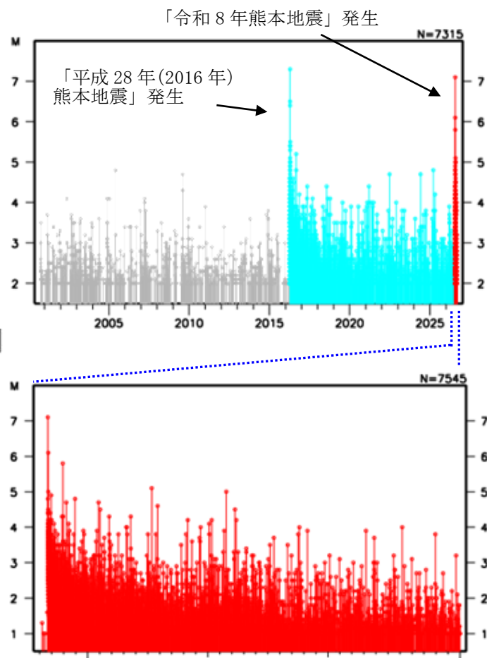
図5 図4の領域a内の地震活動経過図
