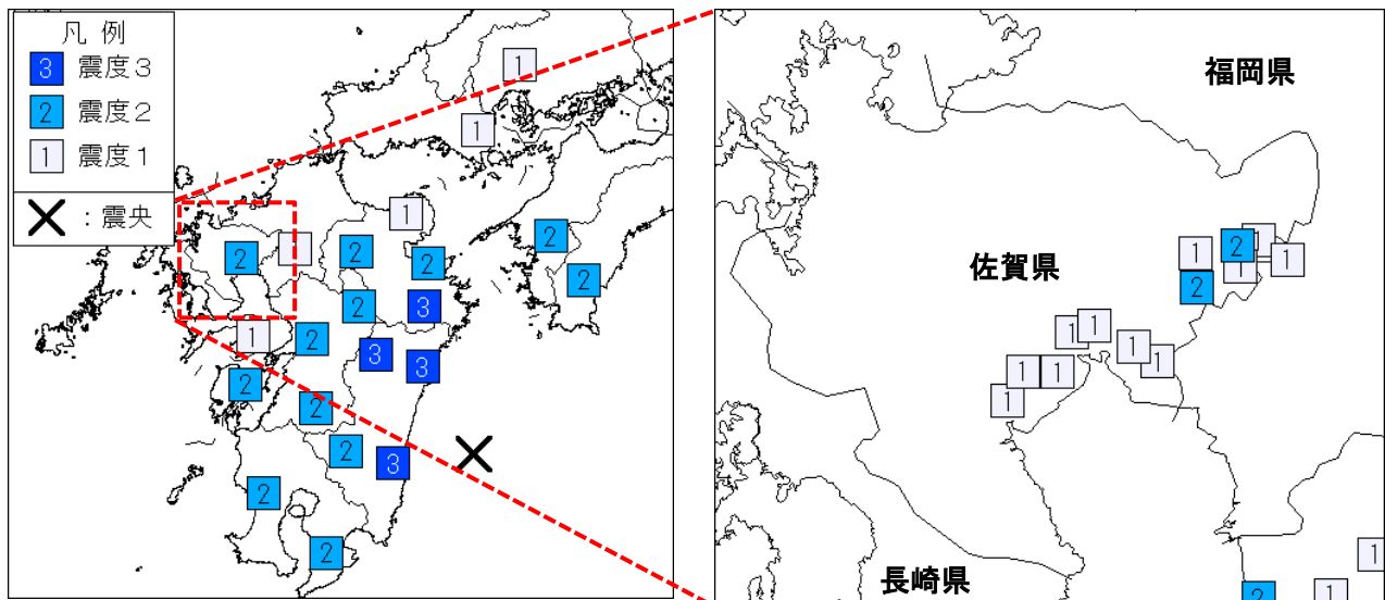
図 6 震度分布図（左図は地域別、右図は観測点別）
