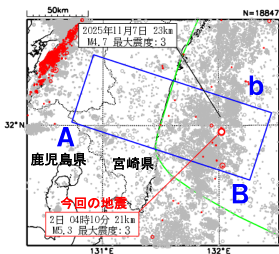
図 7 震央分布図
