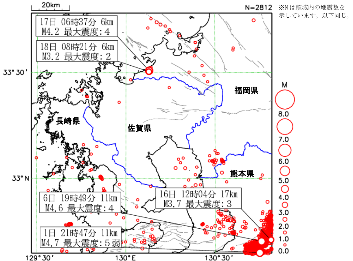
図 1 震央分布図 (2026 年 8 月 1 日～31 日、深さ 30km 以浅、M ≥ 0.0) 灰色の線は地震調査研究推進本部の長期評価による活断層を示しています。
