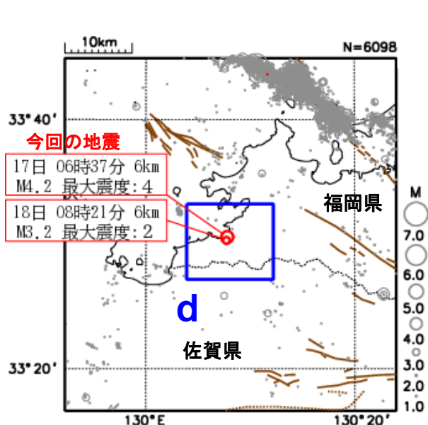
図11 震央分布図
