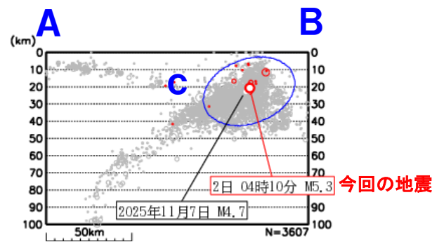
図 8 図 7 の領域 b 内の断面図 (A-B 投影)
