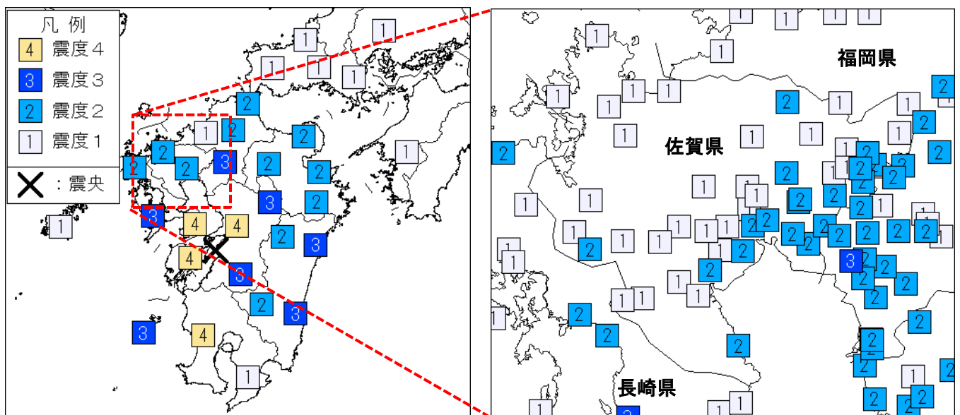
図 3 震度分布図 （左図は地域別、右図は観測点別） 6 日 07 時 59 分 M5.1 (8 月の地震活動の最大規模の地震)
