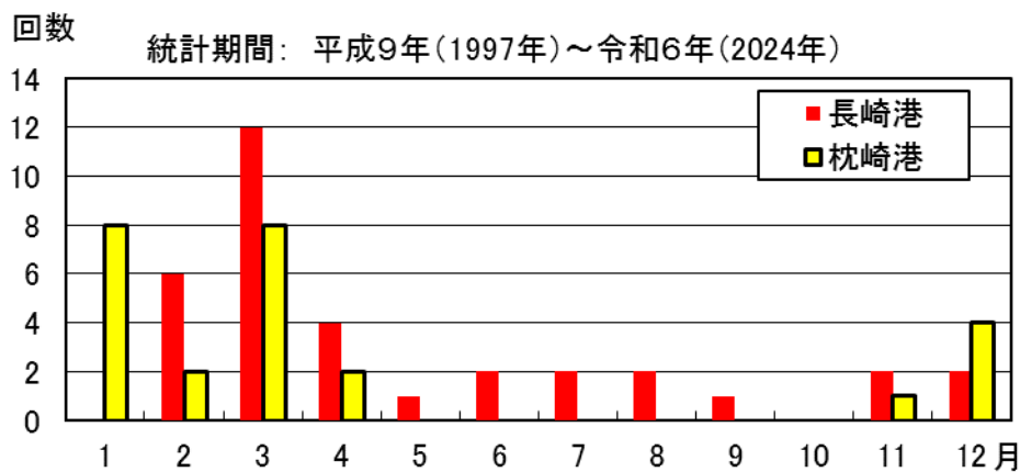
図2 「あびき」の月別発生回数 （長崎港（長崎県）と枕崎港（鹿児島県）における100センチ以上の回数）
