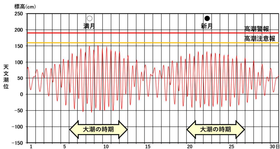
図3 唐津における2025年9月（1時間ごとの）の天文潮位
