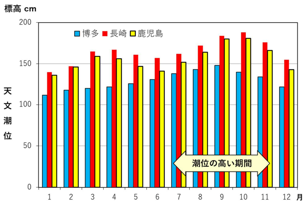
図2 博多・長崎・鹿児島における 2025 年の各月最高の天文潮位
