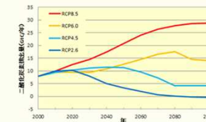
それぞれのRCPシナリオの二酸化炭素排出量の想定(炭素重量換算)。
