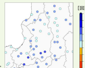
1時間降水量30mm以上の年間発生回数(分布図)
