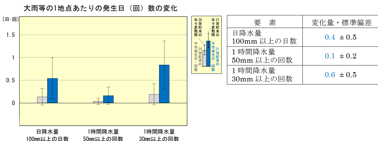
図 5.3.5-2 留萌地方の大雨等の年間発生日（回）の変化及び付表（単位：日・回）【バイアス補正済み】 青色の棒グラフは将来気候における発生日（回）数（4 メンバーの平均）を、灰色の棒グラフは現在気候の発生日（回）数を、細い縦線は現在気候と将来気候の年々変動の幅（標準偏差）を示している。付表は将来気候における変化量と年々変動の幅を「変化量±標準偏差」で示し、その変化量が信頼度水準 90%で有意に増加する場合は青字としている。 ※地域によっては地域内の変化量が大きく異なる場合がありますが、ここでは地域全体の平均的な発生日（回）数であることを注意してください。
