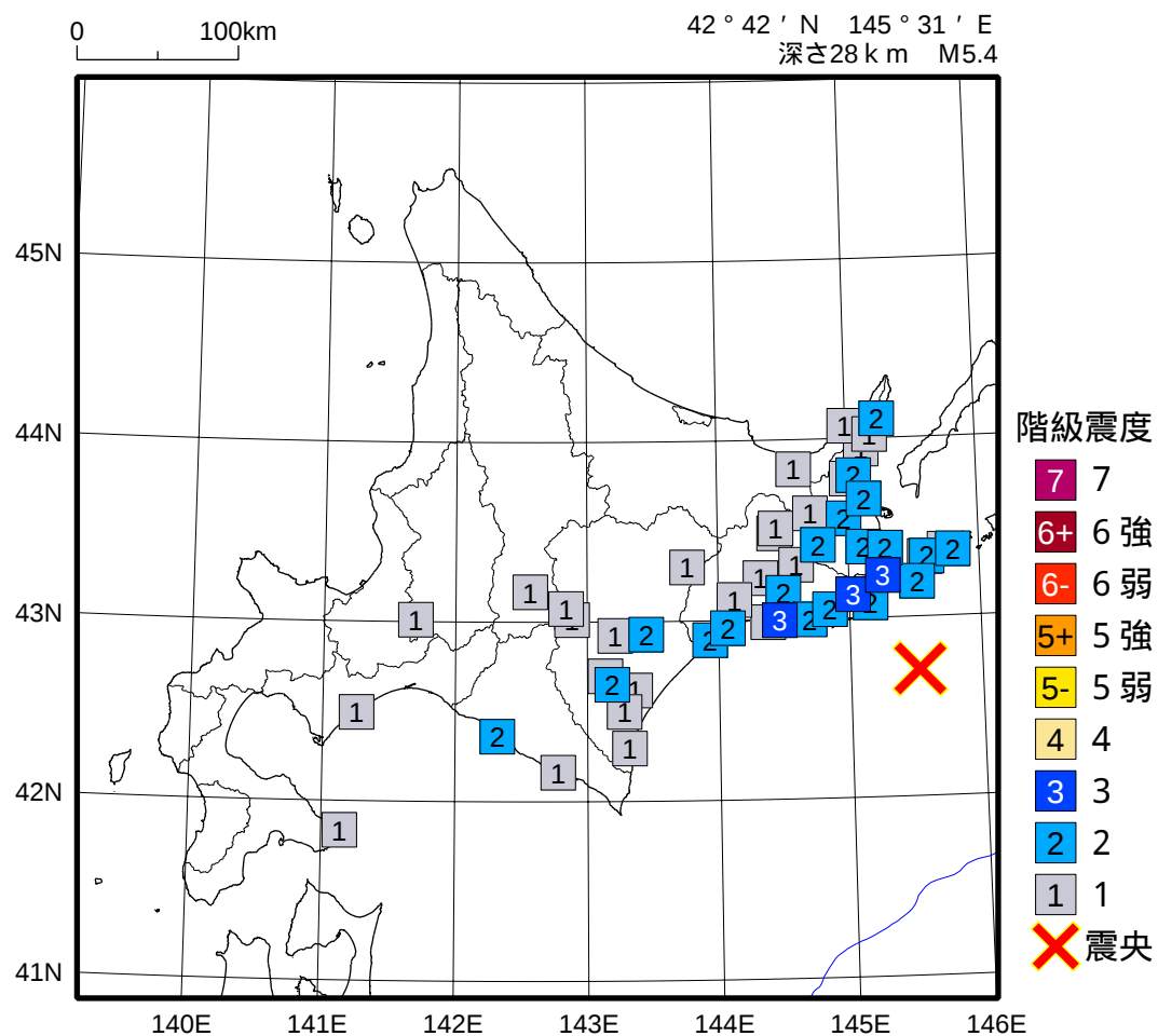
2024年 7月21日13時27分 釧路沖の地震の震度分布図
