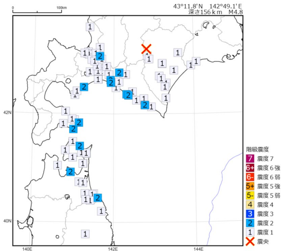
図4 震度分布図の例
