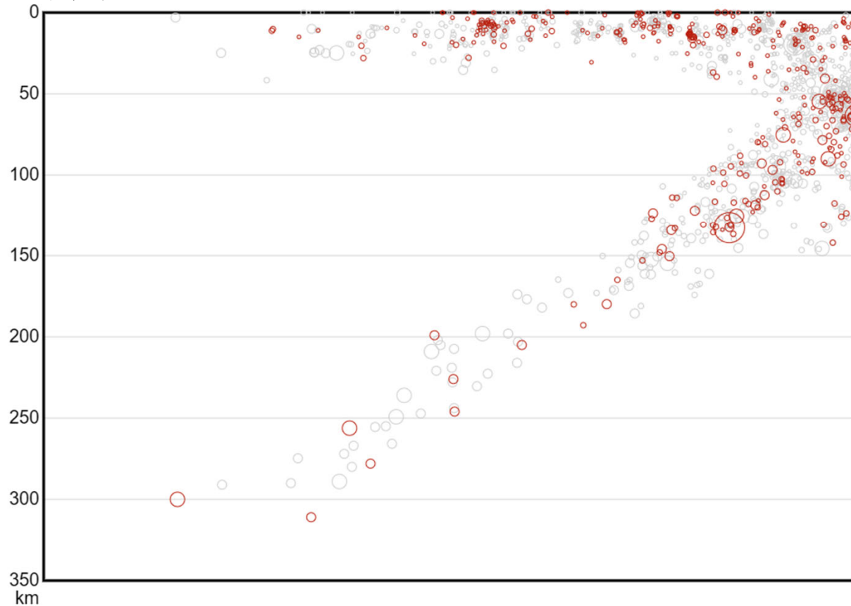
断面図
