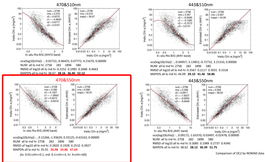
図 JAXA 村上氏による、中心波長を変化させたクロロフィル a 濃度推定精度の変化シミュレーション。0.47 \mu\text{m} と 0.55 \mu\text{m} の組み合わせがベストであることを示している。
