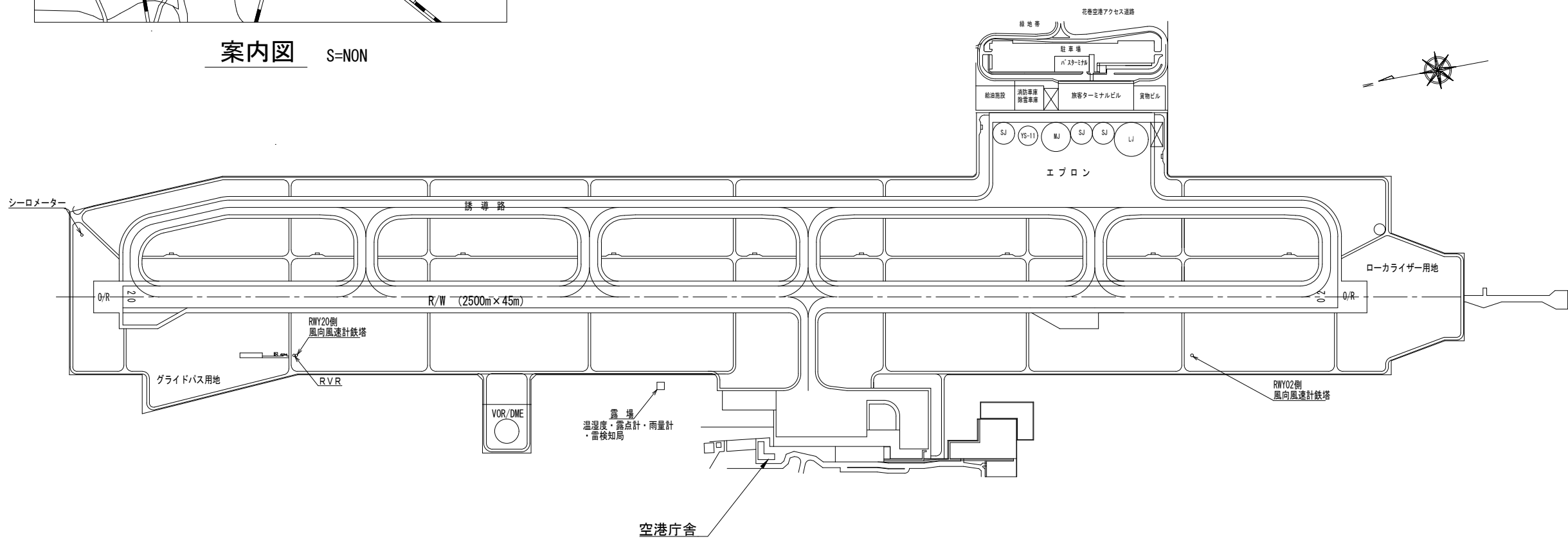
空港平面図 S=1/10000
