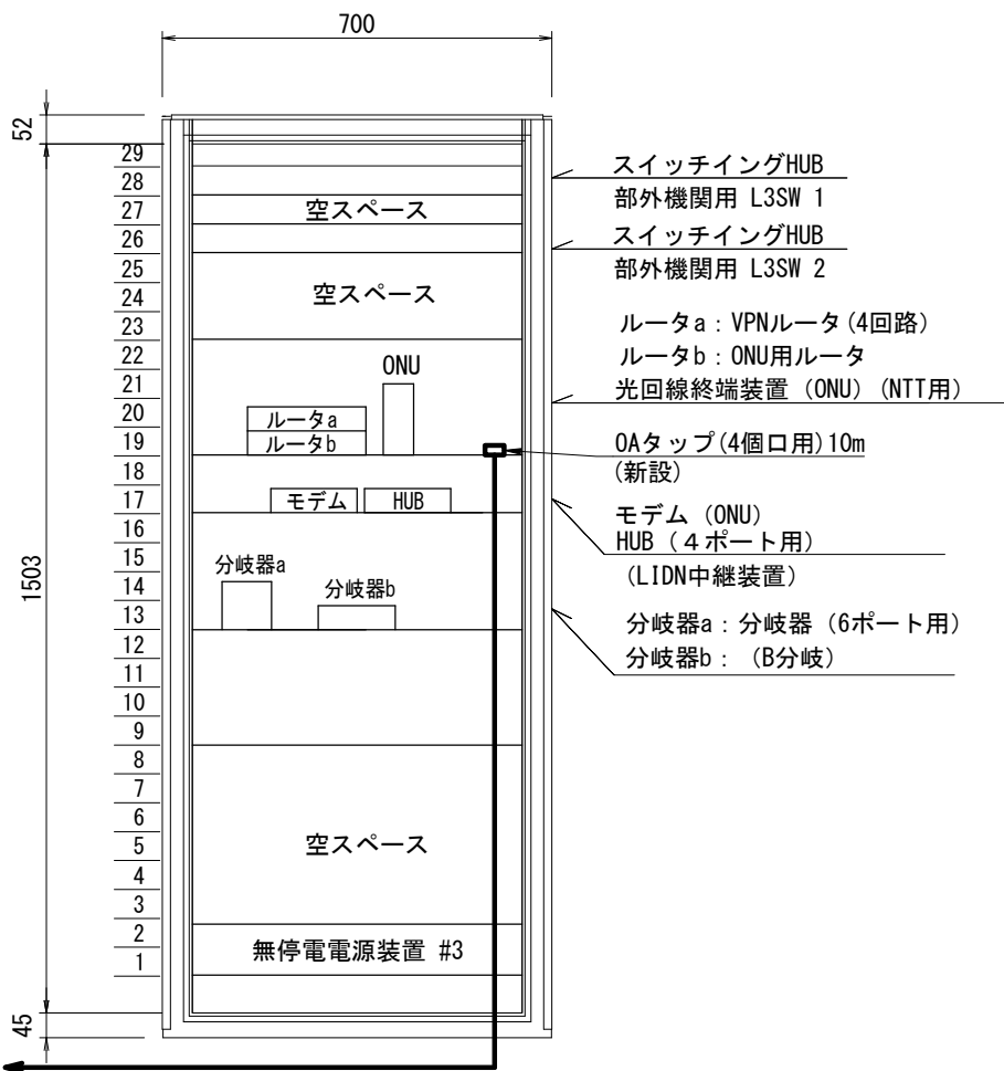
内部実装図（正面）
