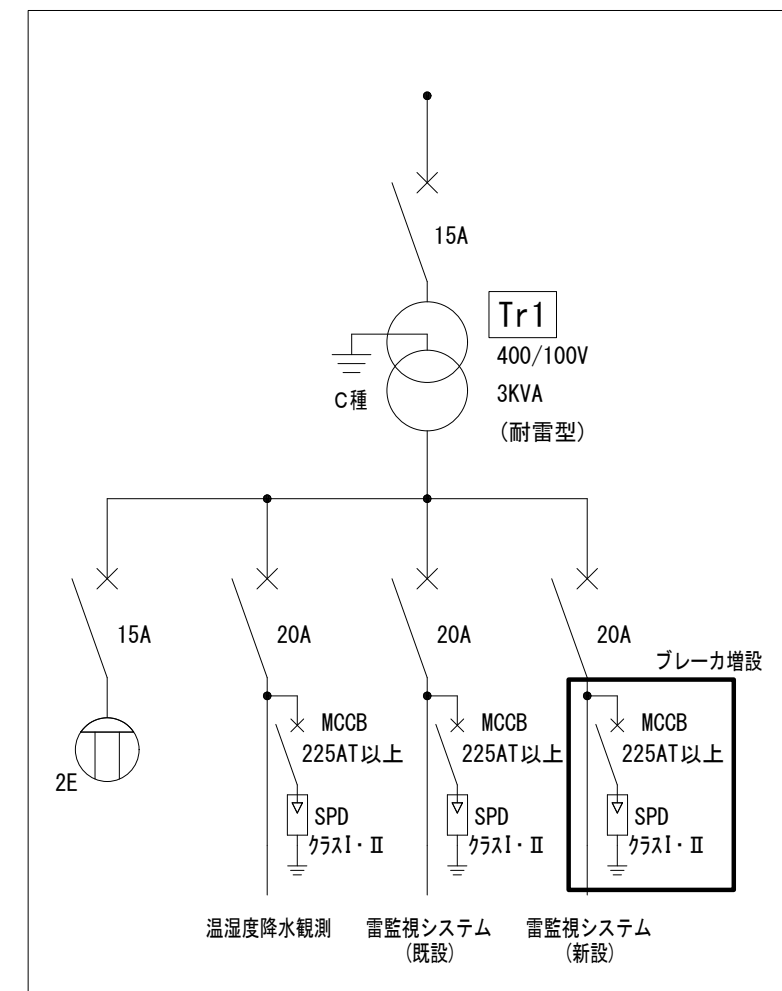
M I D 露場屋外分電盤
