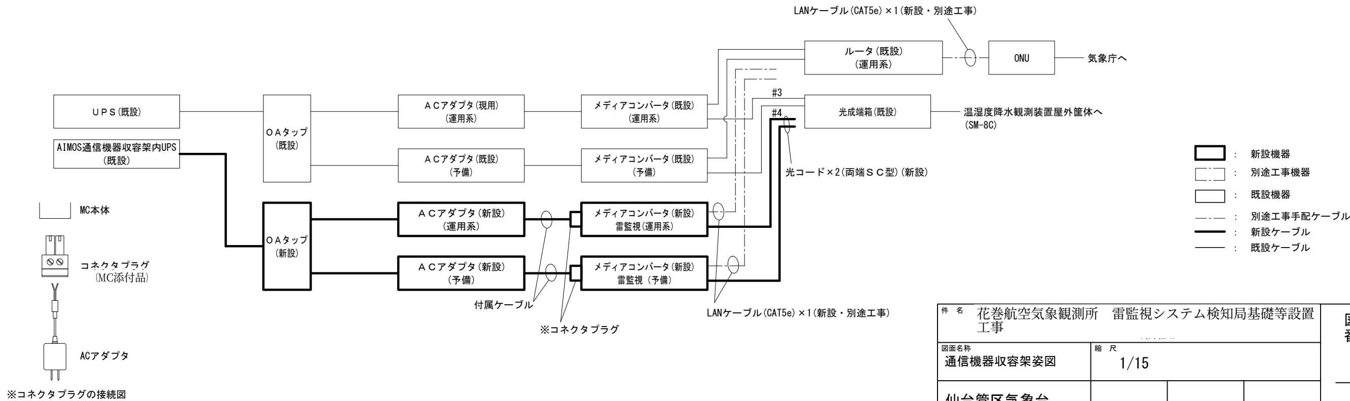
雷監視システム用配線系統図
