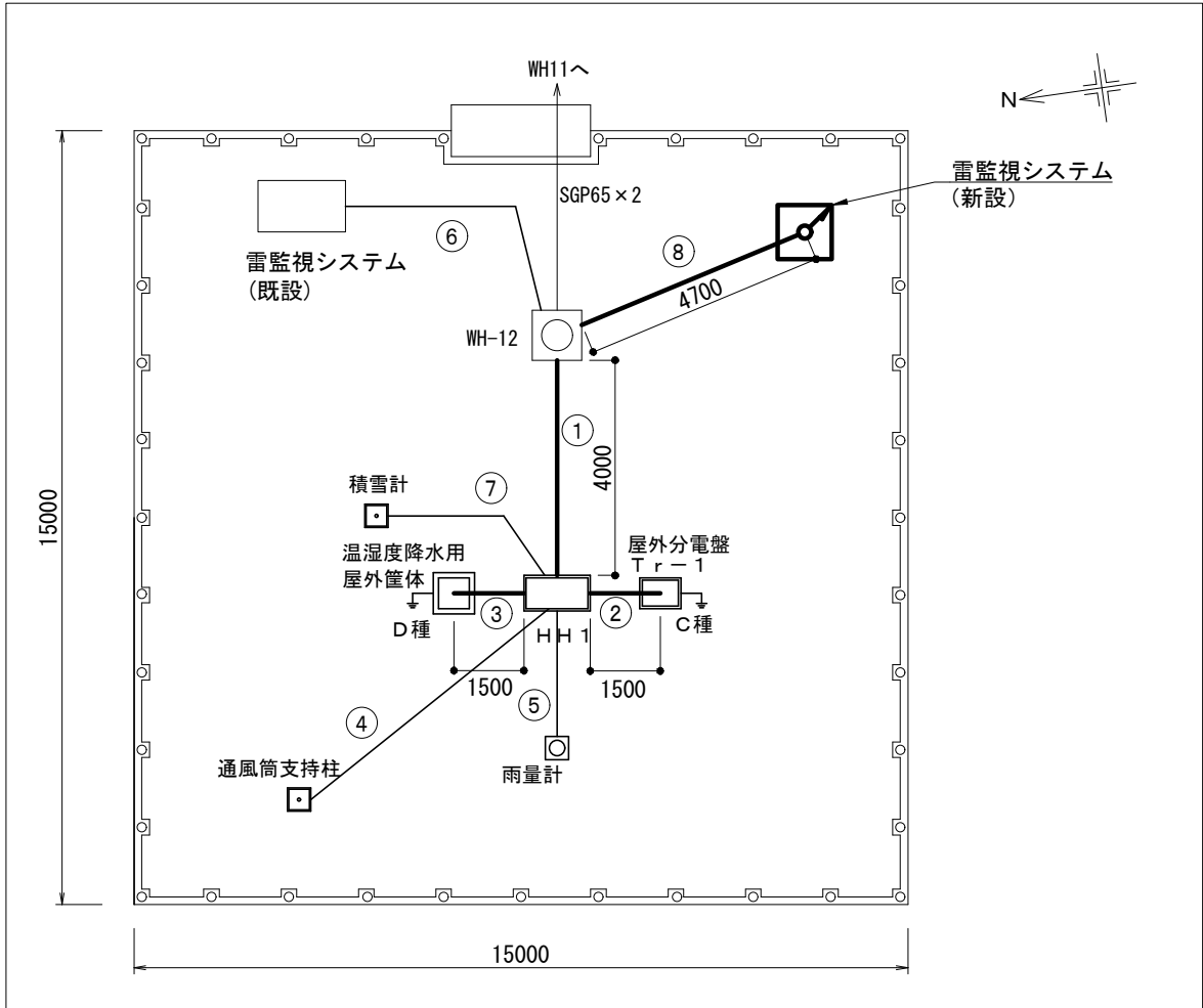
露場側 屋外配線図 S=1/150
