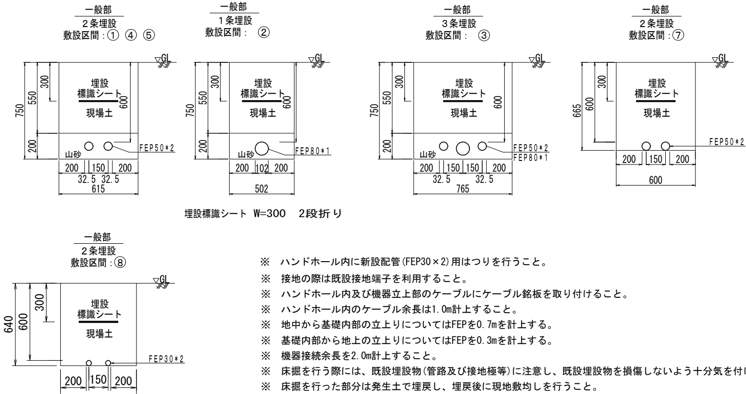
管路掘削断面図 S=1/30
