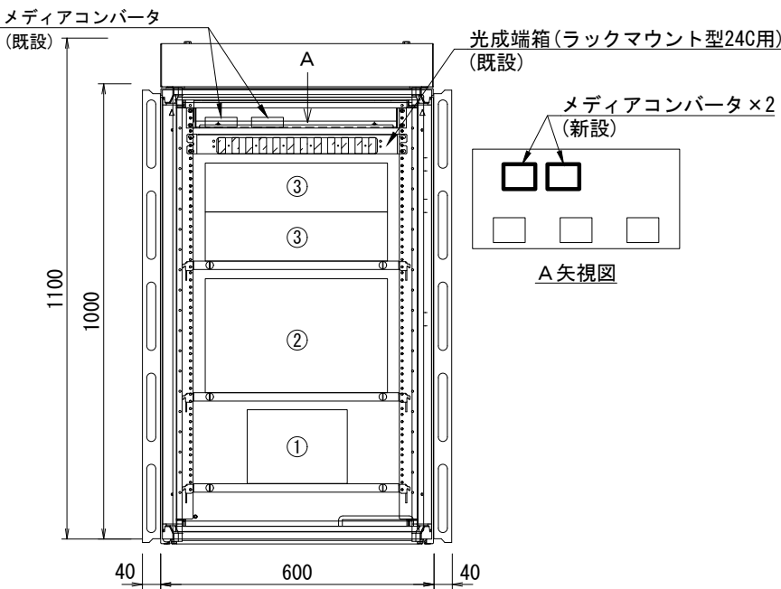
温湿度降水観測用屋外筐体実装図
