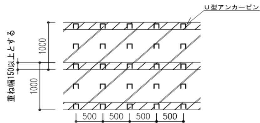
U型アンカーピン施工例
