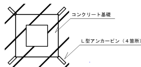
L型アンカーピン施工例
