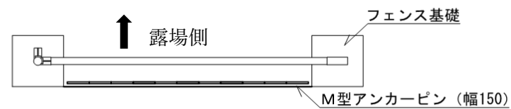
M型アンカーピン施工例
