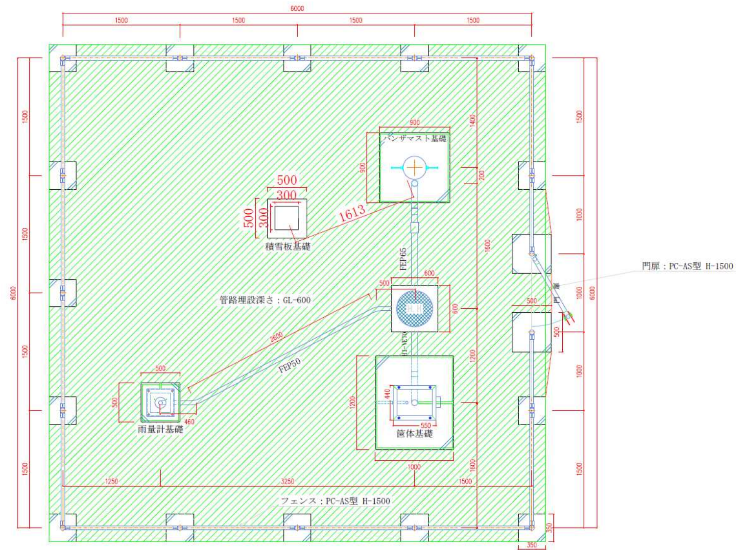
露場 配置図 (防草シート敷設)
