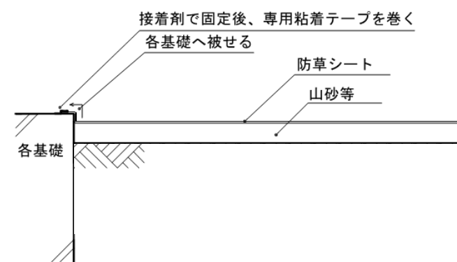
防草シート敷設時の断面図
