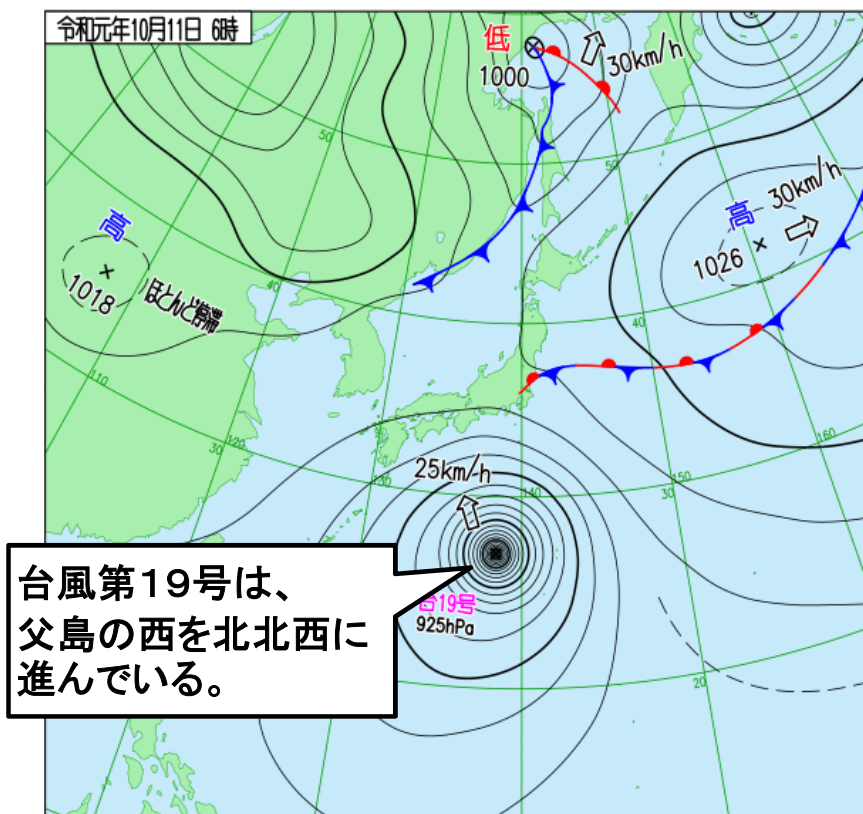
11日06時 天気図
