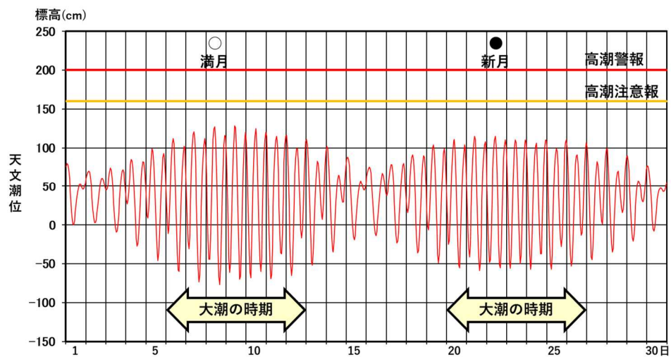
図3 下関（弟子松）における2025年9月（1時間ごとの）の天文潮位
