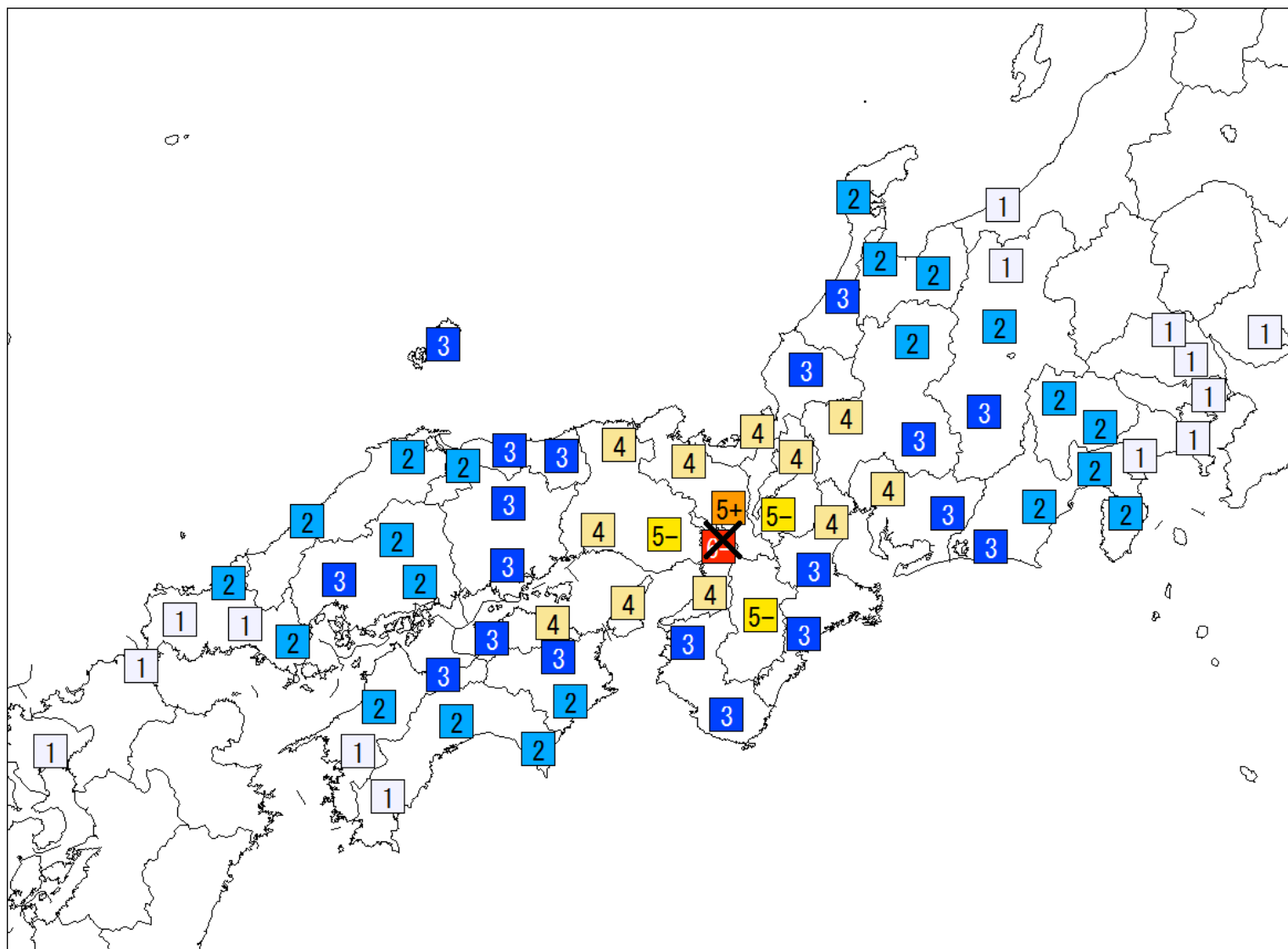
地域震度分布図（×は震央を表す）
