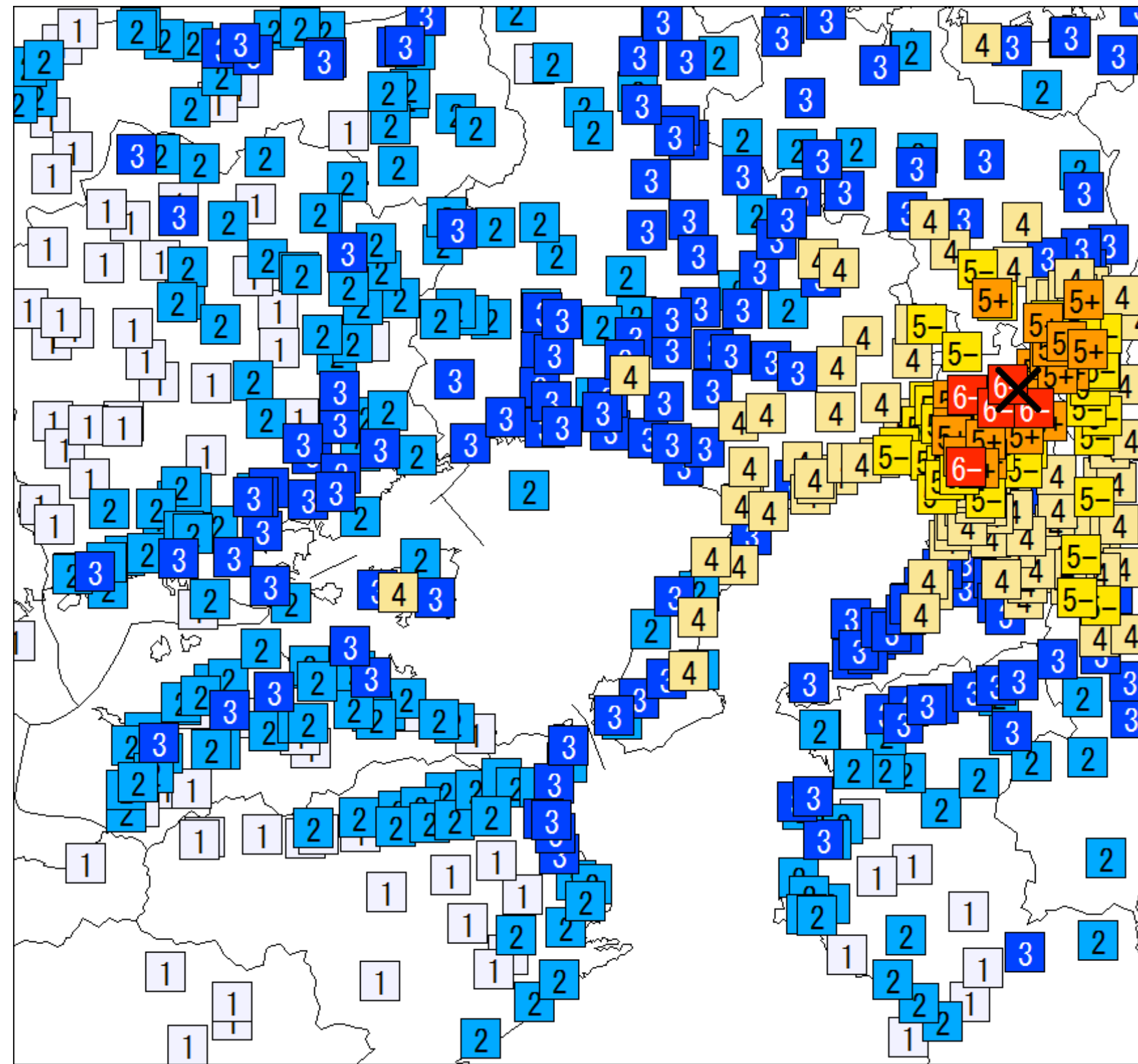
観測点震度分布図（×は震央を表す）
