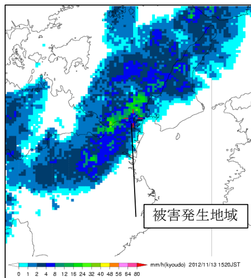
レーダー画像（11月13日15時20分）
