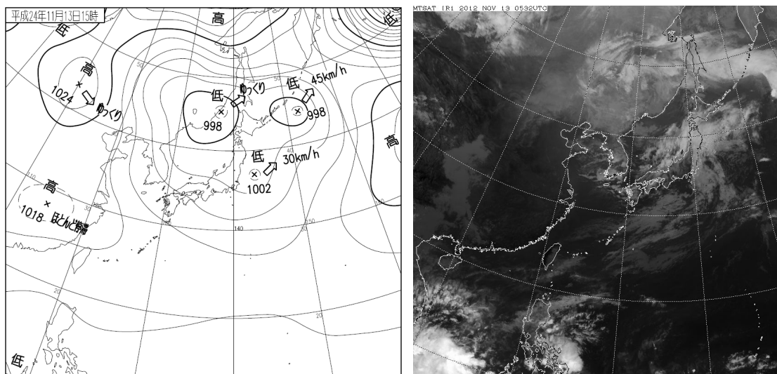
11月13日15時の地上天気図（左）と気象衛星赤外画像（右）
