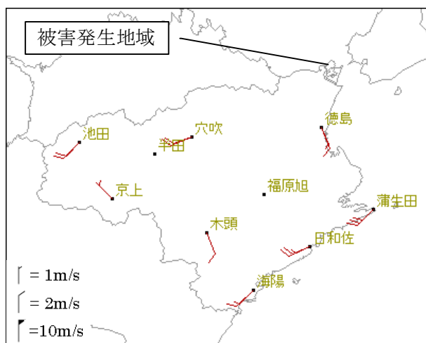
アメダス地点における前10分平均風向風速分布図（11月13日15時20分）
