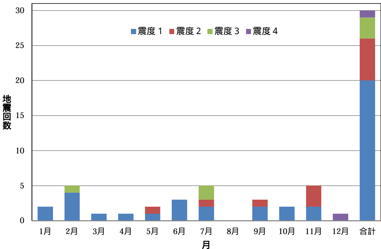
徳島県内月別最大震度別地震回数グラフ（2021年）
