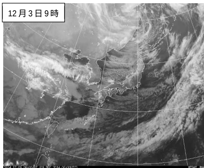
地上天気図および気象衛星「ひまわり7号」赤外画像
