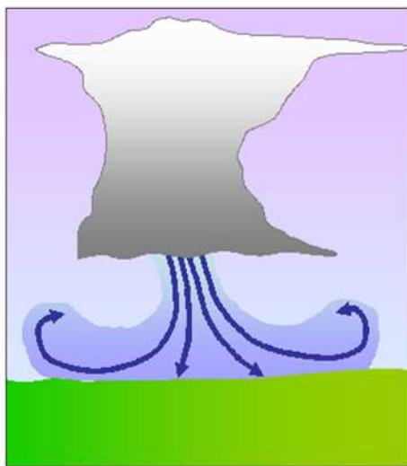
ダウンバーストのイメージ図
