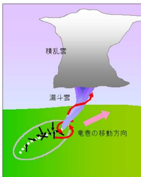
竜巻とその被害の様子
