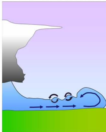
ガストフロントのイメージ図
