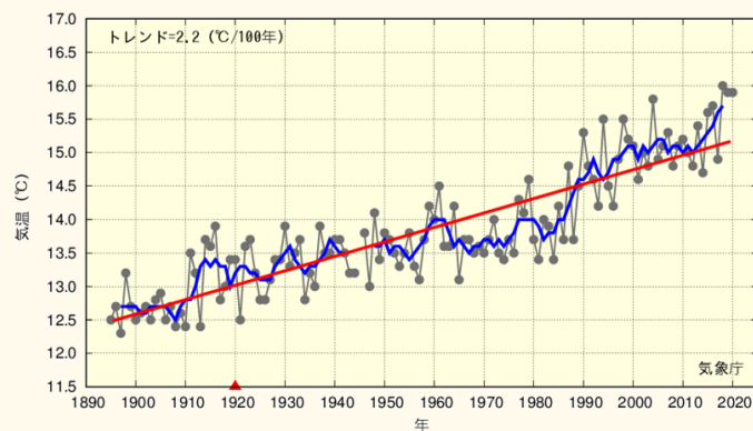
甲府(甲府市)の年平均気温
