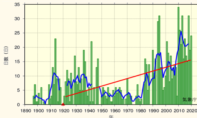
甲府(甲府市)の年間猛暑日日数
