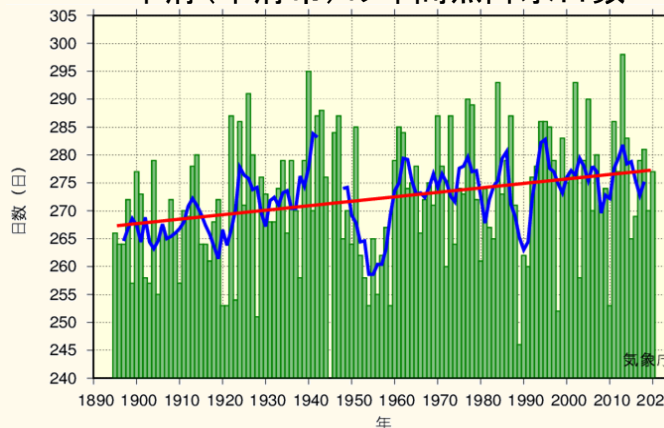
甲府(甲府市)の年間無降水日数
