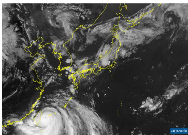
7 月 24 日 12 時の地上天気図（左）と気象衛星赤外画像（右）
