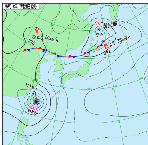
7 月 24 日 12 時の地上天気図（左）と気象衛星赤外画像（右）
