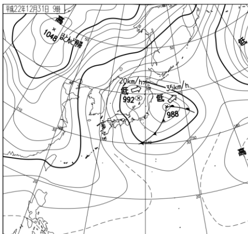
12月31日9時の地上天気図（左） 気象衛星赤外画像（右）
