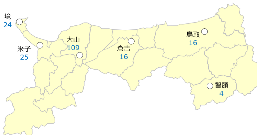
1 月 1 日 12 時の県内観測地点の積雪量
