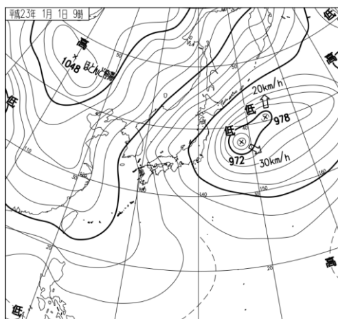
1月1日9時の地上天気図（左）と気象衛星赤外画像（右）
