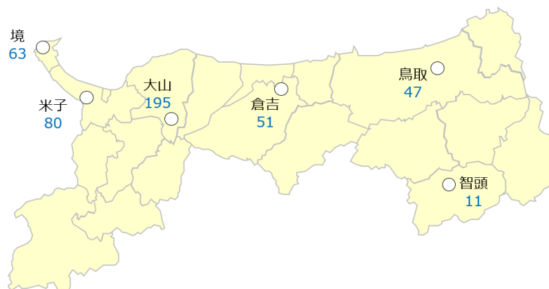
1 月 1 日 12 時の県内観測地点の積雪量
