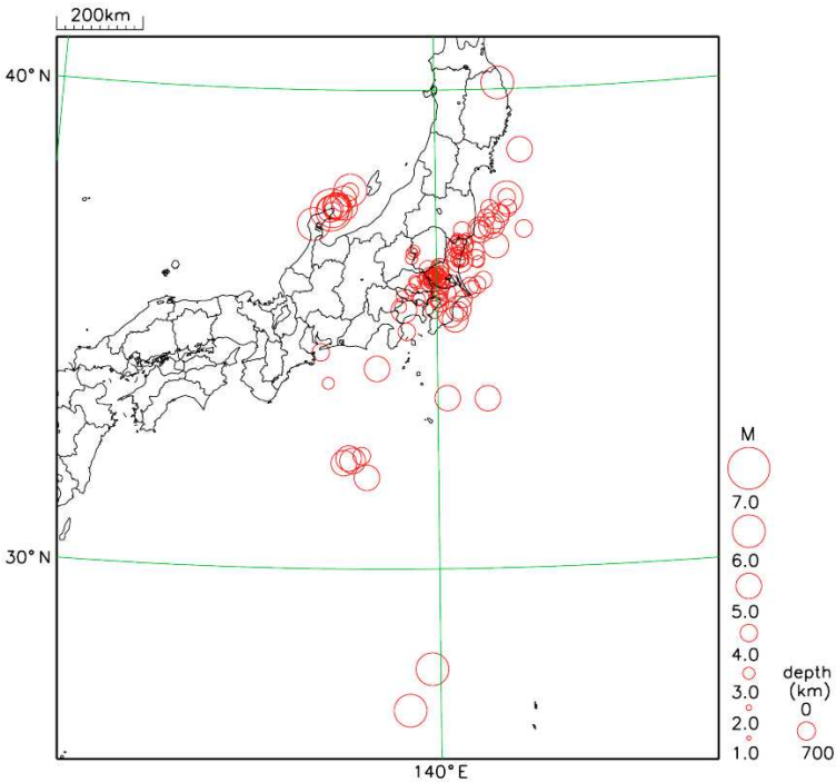
○ 2024 年に栃木県内で震度を観測した地震の震央分布図
