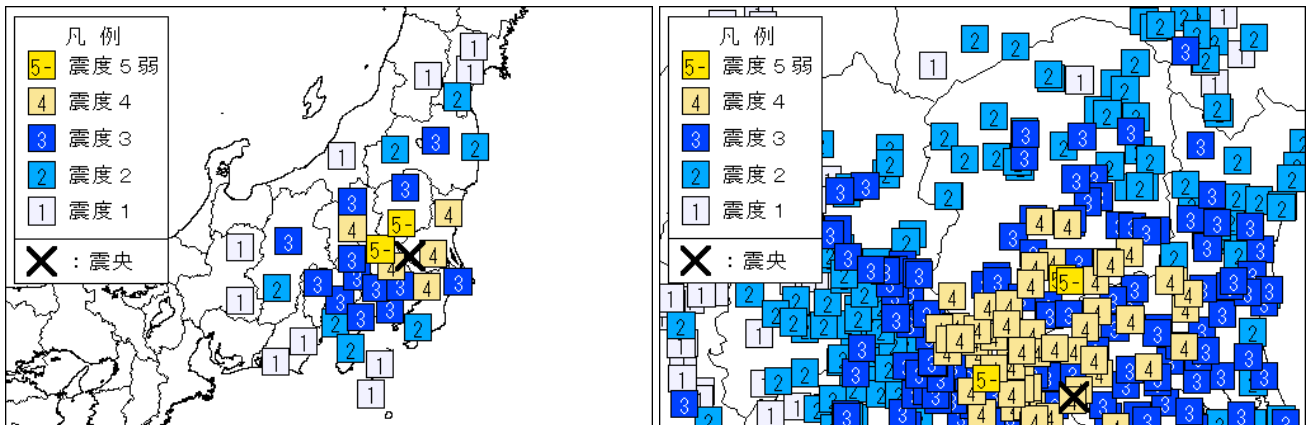
2024年3月21日9時8分 茨城県南部の地震 左図：地域震度 右図：地点震度
