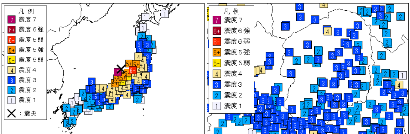
2024年1月1日16時10分 石川県能登地方の地震 左図：地域震度 右図：地点震度
