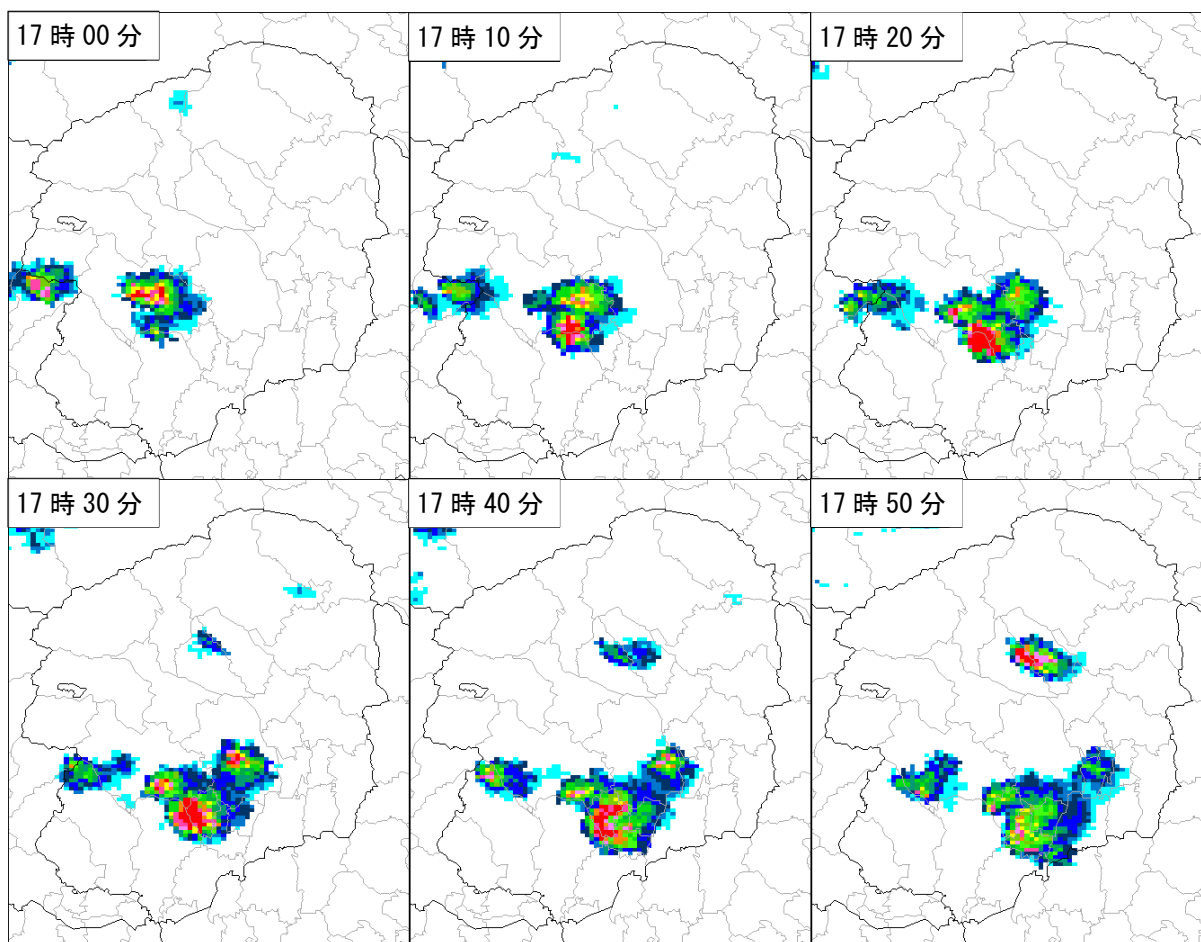
8月15日17時00分から10分毎のレーダー画像
