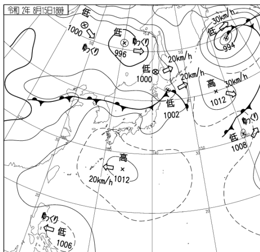
8月15日18時の地上天気図（左）と気象衛星赤外面像（右）
