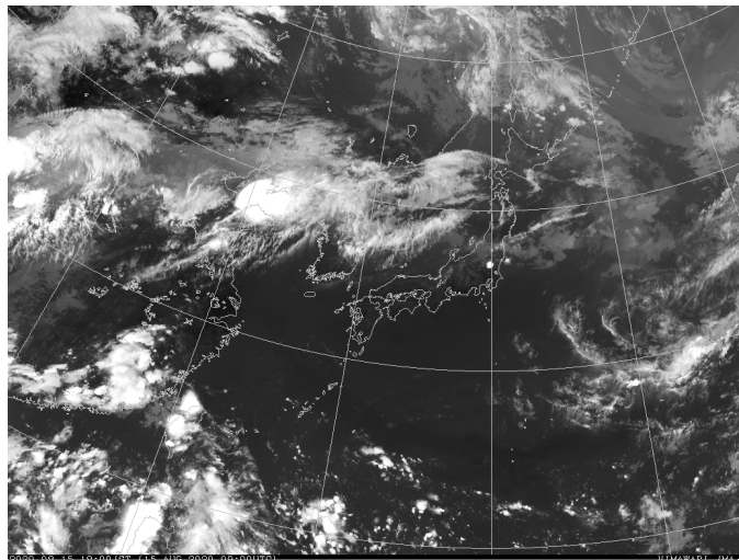
8月15日18時の地上天気図（左）と気象衛星赤外面像（右）
