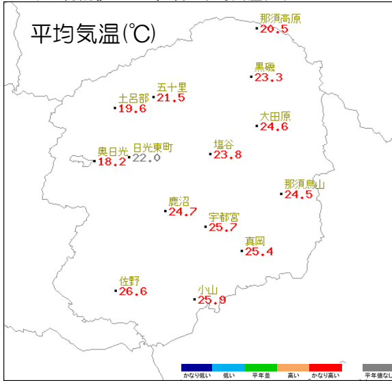
アメダス月別値 2023年9月 平均気温(°C)
