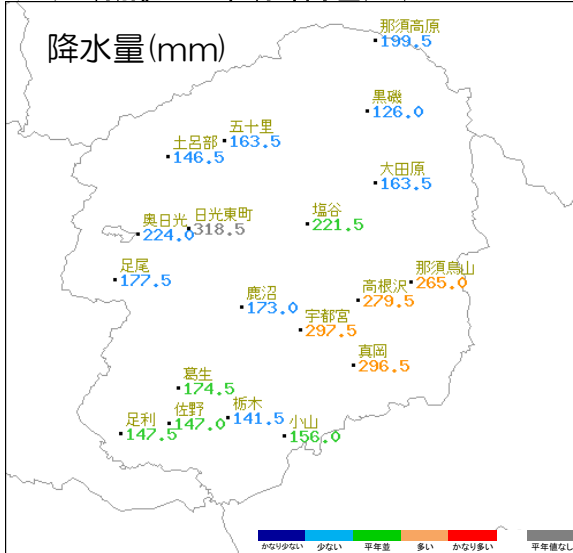
アメダス月別値 2023年9月 降水量(mm)
