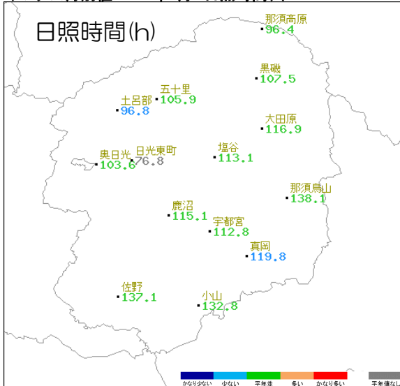
アメダス月別値 2023年9月 日照時間(h)
