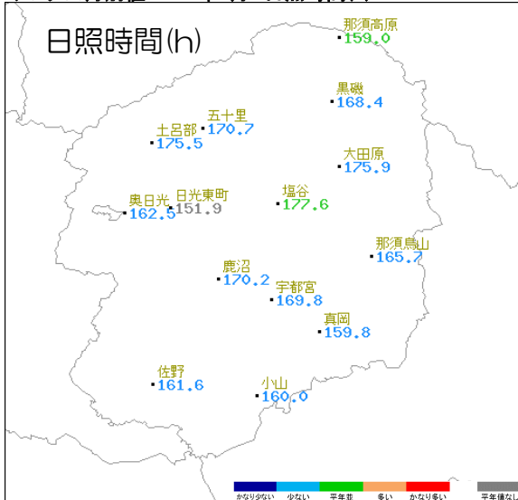
アメダス月別値 2024年4月 日照時間(h)
