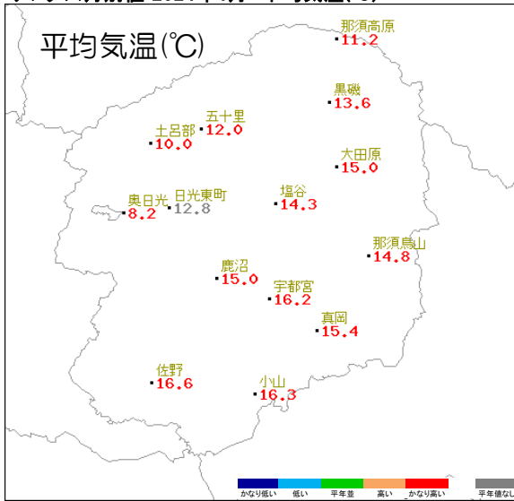
アメダス月別値 2024年4月 平均気温(°C)
