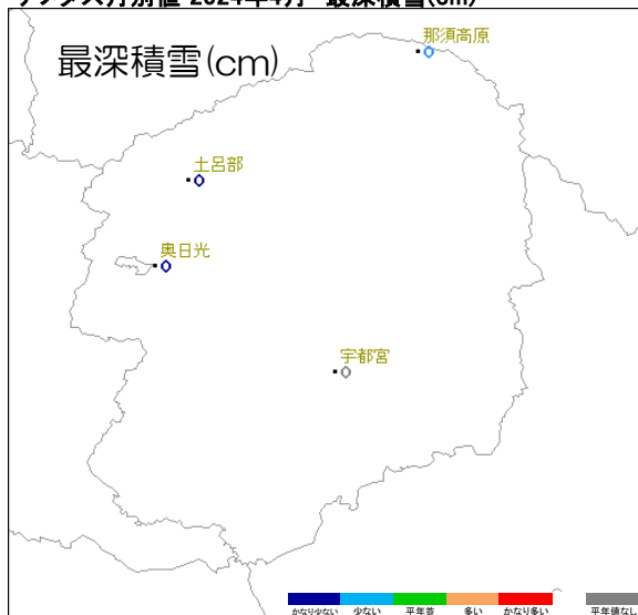
アメダス月別値 2024年4月 最深積雪(cm)
