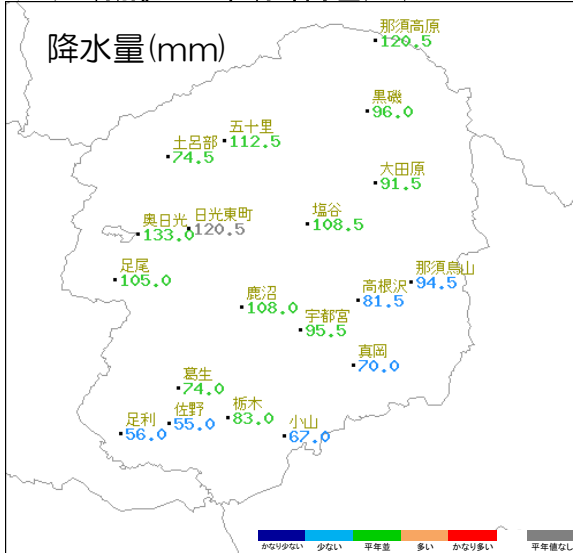
アメダス月別値 2024年4月 降水量(mm)
