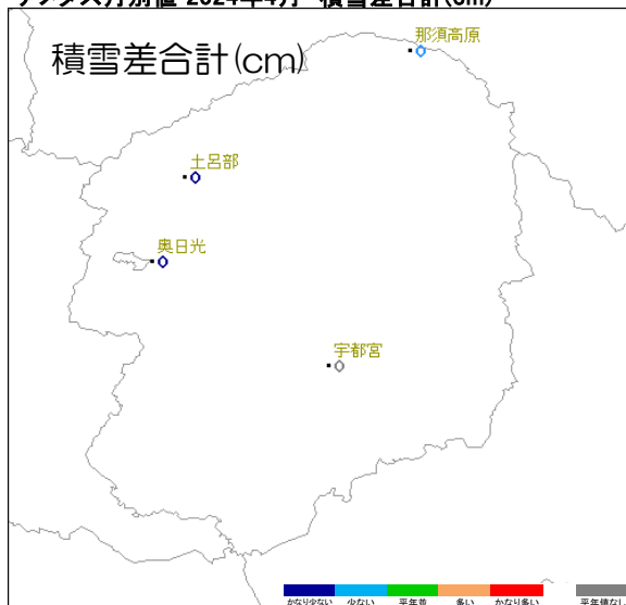
アメダス月別値 2024年4月 積雪差合計(cm)
