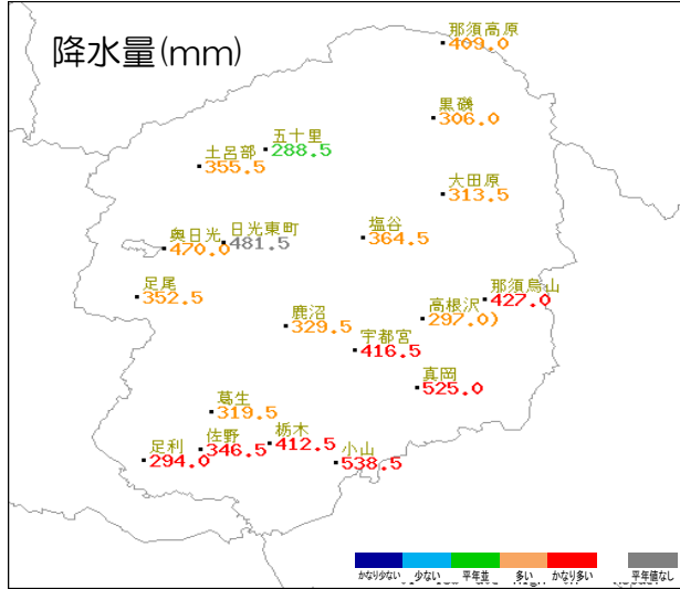
アメダス月別値 2026年9月 降水量(mm)
