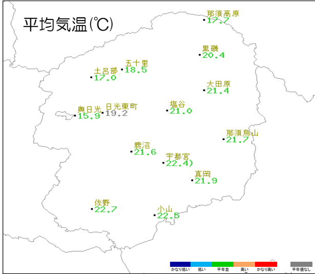
アメダス月別値 2026年9月 平均気温(℃)
