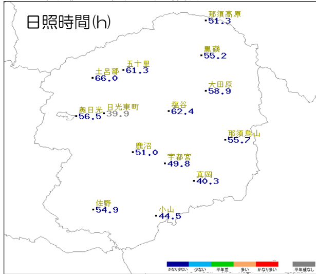
アメダス月別値 2026年9月 日照時間(h)
