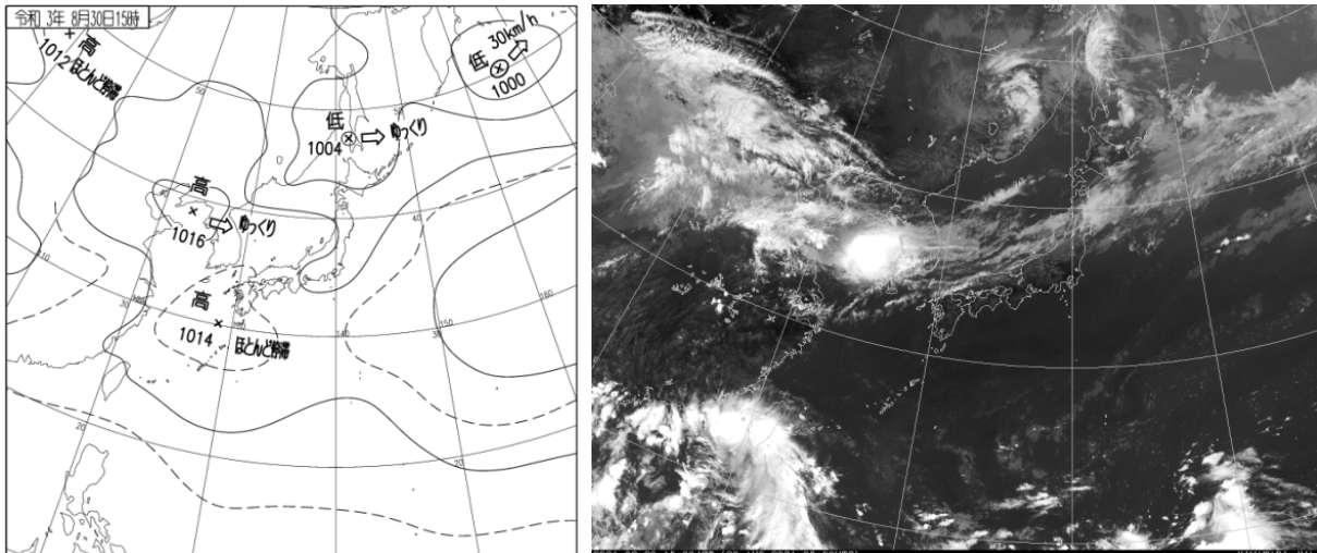
8月30日15時の地上天気図（左）と気象衛星赤外面像（右）
