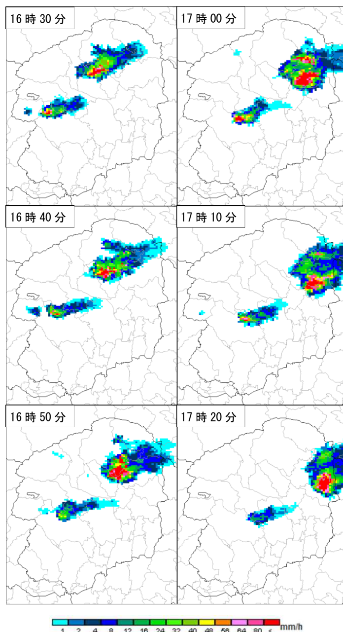
8月30日16時30分から10分毎のレーダー画像
