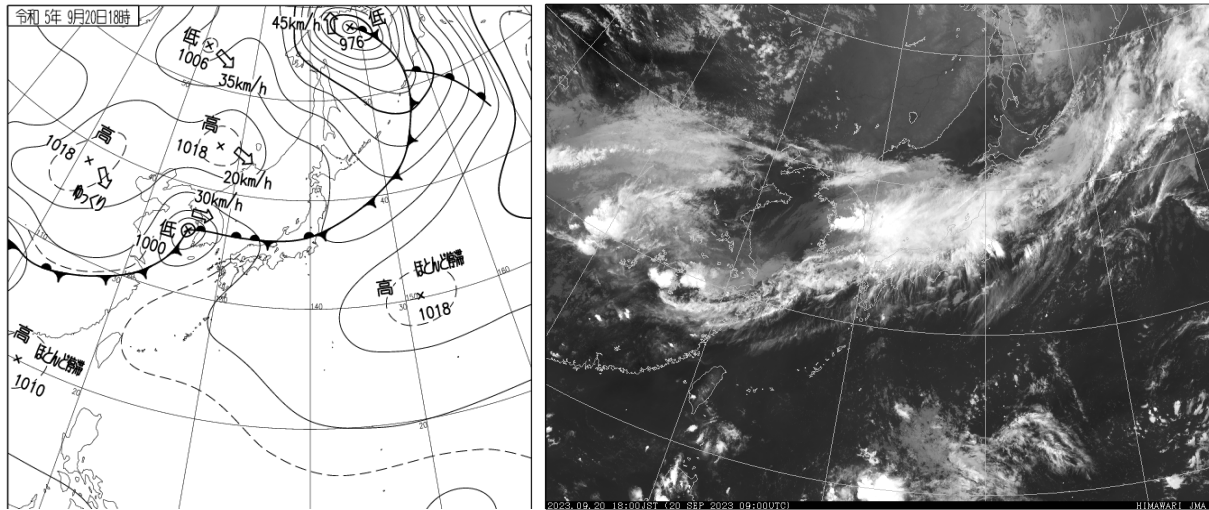
9月20日18時の地上天気図（左）と気象衛星赤外面像（右）
