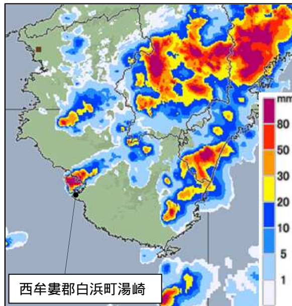
レーダー画像 (8 月 25 日 14 時 30 分)
