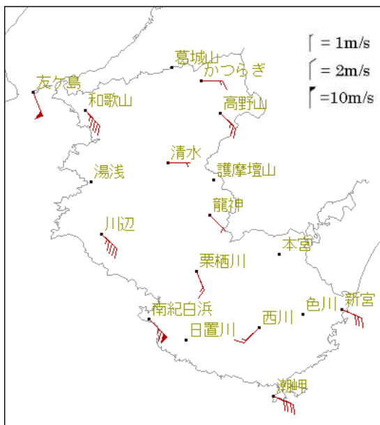
アメダス地点における風向風速分布図 (8 月 25 日 14 時 00 分)
