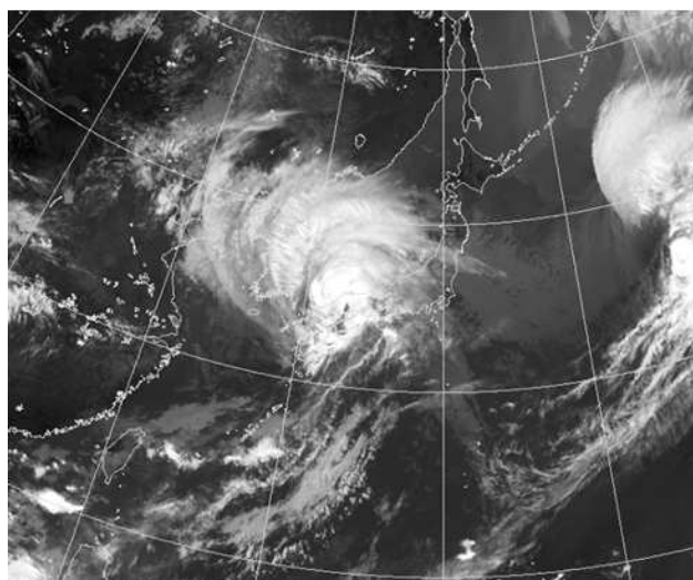
8 月 25 日 12 時の地上天気図（左）と気象衛星赤外画像（右）
