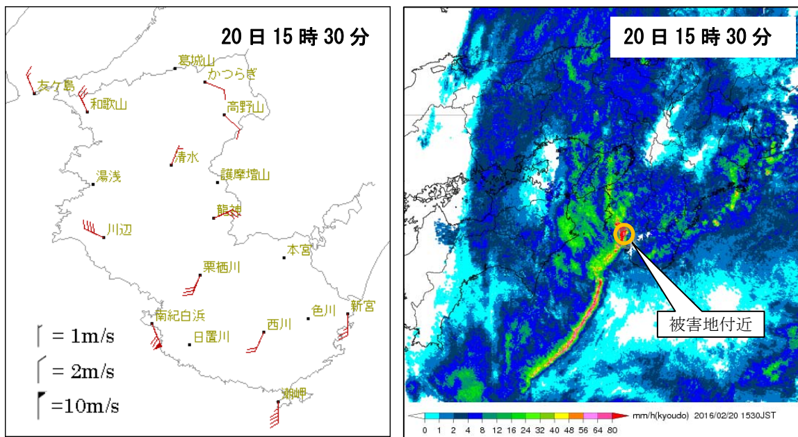
アメダス地点における風向・風速分布図 「・」のみの地点では風の観測を行っていない。
