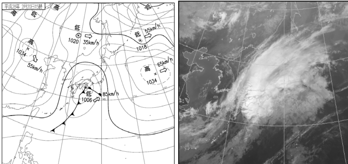
2 月 20 日 15 時の地上天気図（左）と気象衛星赤外画像（右）
