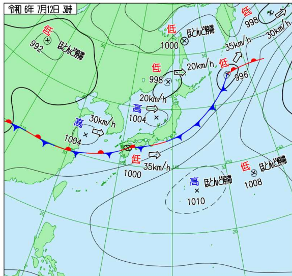
地上天気図(令和6年7月12日03時、09時、15時)
