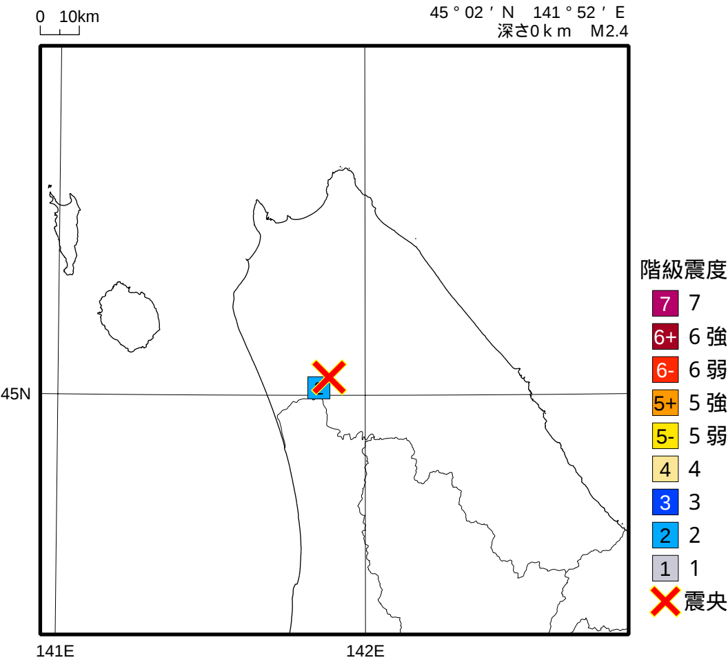
2022年 9月 2日09時09分 宗谷地方北部の地震の震度分布図
