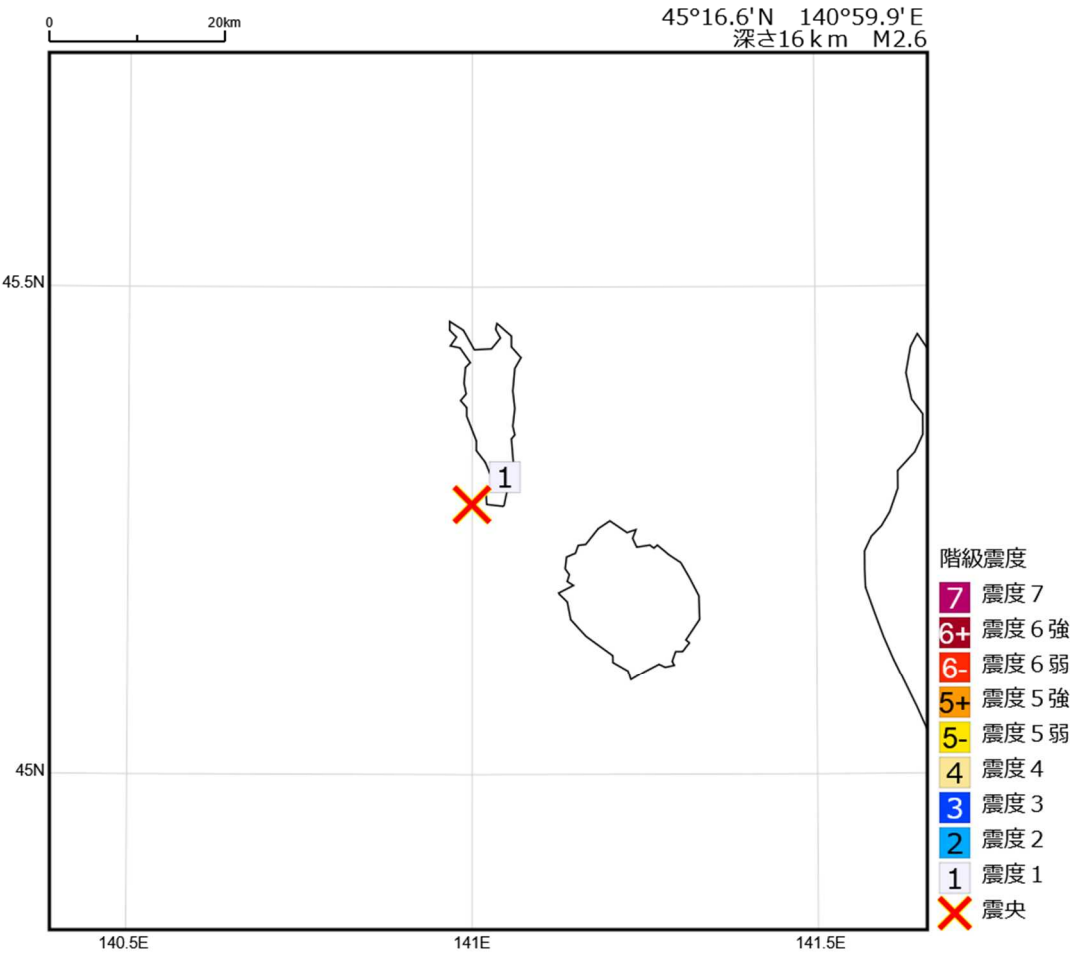
2025年 1月 7日 23時07分 北海道北西沖の地震の震度分布図
