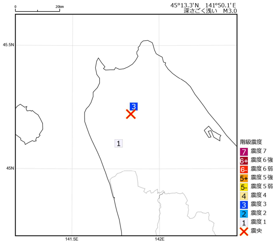
2025年 3月25日 06時53分 宗谷地方北部の地震の震度分布図
